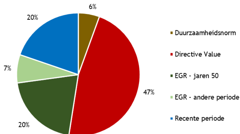
Figuur 2.3. Aandeel van de beoordeelde broedvogelsoorten (soorten zonder gebiedsdoelen, n=162) waarin een bepaald criterium als uitgangspunt diende voor de GRW.
