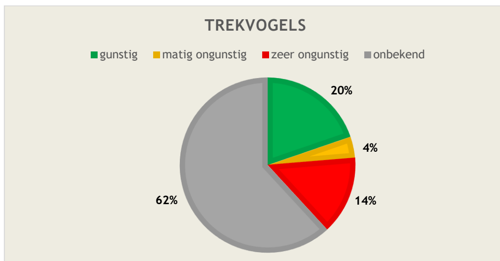
Figuur 5.1. Het aandeel soorten met een gunstige Svl, een matig ongunstige Svl, zeer ongunstige of onbekende Svl (n=152).
