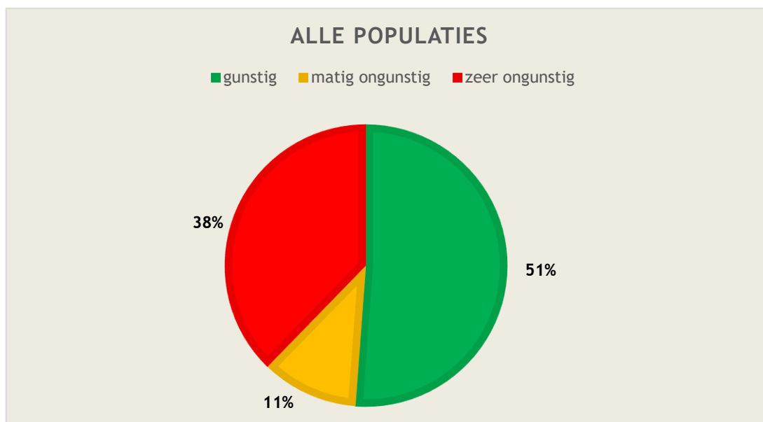
Figuur 7.3. Het aandeel van alle beoordeelde soorten waarover een uitspraak over de SvI kon worden gedaan met een gunstige SvI, een matig ongunstige SvI, zeer ongunstige SvI of onbekende SvI (n=295).
