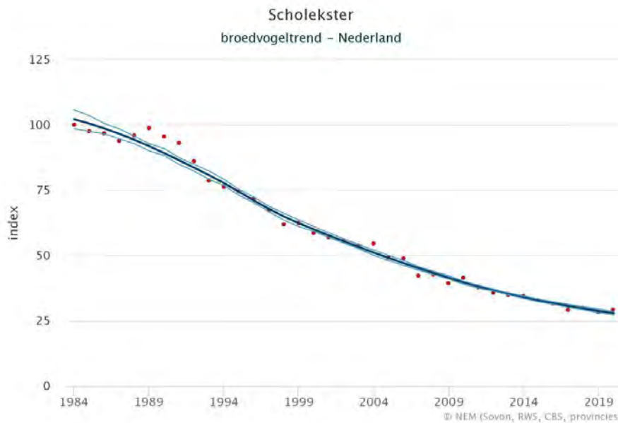
Figuur 4. Trend van Scholekster als broedvogel in Nederland: een voorbeeld van een soort waarvoor de aantallen broedparen, dankzij tellingen in steekproefgebieden, een heel duidelijke trend laten zien.
