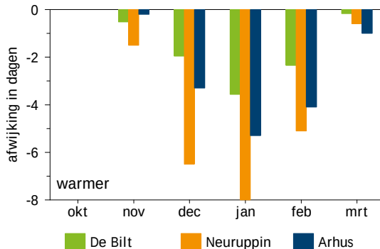
Figuur 3.4. Weeromstandigheden in Noord- en Oost-Europa in 2019/20, afgeleid uit het aantal ijsdagen (max. temperatuur < 0°C) in Arhus (Jutland, Denemarken) en Neuruppin (Brandenburg, Duitsland) (wetteronline.de). Weergegeven is de afwijking in dagen ten opzichte van de waarde in 1982-2004. Ter vergelijking is ook de situatie in De Bilt NL weergegeven. / Weather characteristics in northern (Arhus, Denmark) and eastern (Neuruppin, eastern Germany) Europe in 2019/20. Shown are the number of days with maximum temperatures < 0°C, expressed as the deviation in days from averages in 1982-2004. The Netherlands (De Bilt) is shown for comparison.
