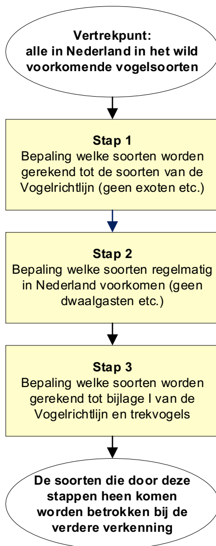
Figuur 2.1. Stappen om de soorten te bepalen waarvoor mogelijk belangrijke gebieden geïdentificeerd worden. De stappen worden hierna verder toegelicht.
