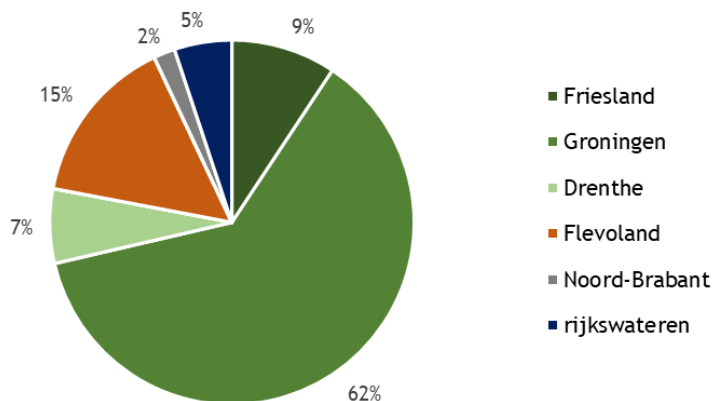
Figuur 4. Aanwezigheid van de Grauwe Kiekendief als broedvogel in de afgelopen zes jaar (2015-2020) per provincie (exclusief rijkswateren) en in de rijkswateren. De rijkswateren zijn gedefinieerd als het voortouwgebied van RWS.
